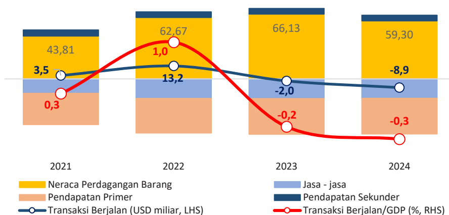
Grafik 13. Transaksi Berjalan, 2021 – 2024 (USD miliar)
