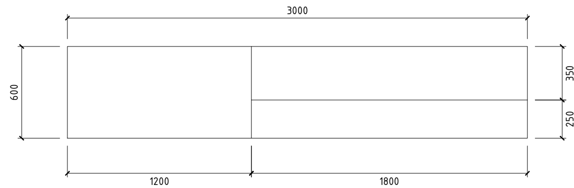
KP - KABINET PANTRY TAMPAK ATAS SKALA 1 : 25
