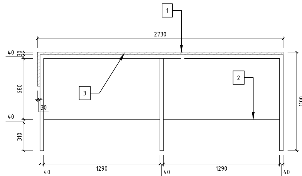
MB - MEJA BAR TAMPAK DEPAN SKALA 1 : 25
