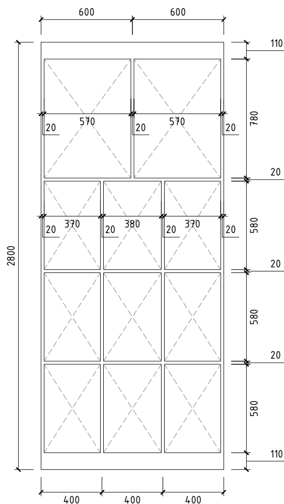
LK 1 – LOKER PENYIMPANAN 1 TAMPAK DEPAN (TERBUKA) SKALA 1 : 25
