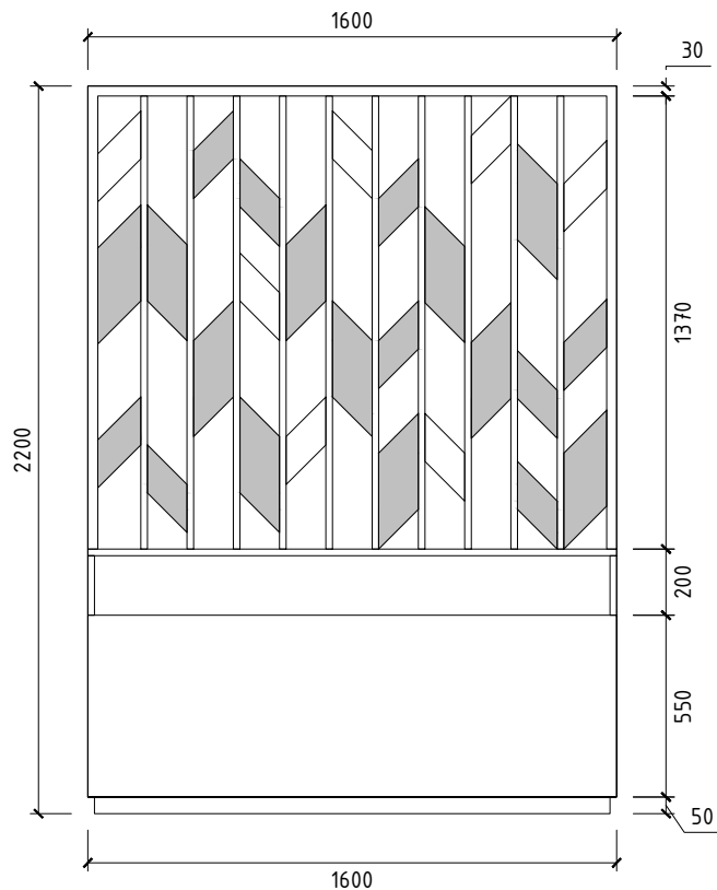
PB - PLANTER BOX TAMPAK DEPAN SKALA 1 : 25
