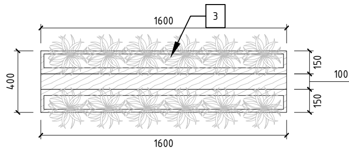
PB - PLANTER BOX TAMPAK ATAS SKALA 1 : 25
