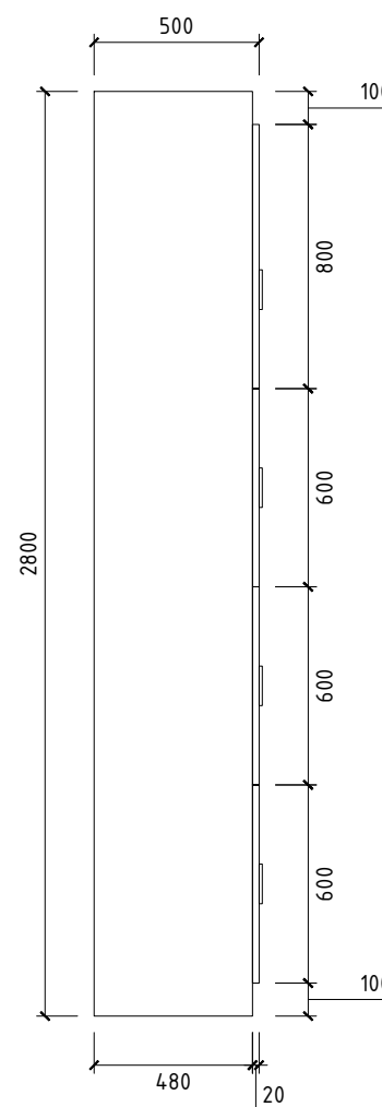
LK 1 – LOKER PENYIMPANAN 1 TAMPAK SAMPIING SKALA 1 : 25
