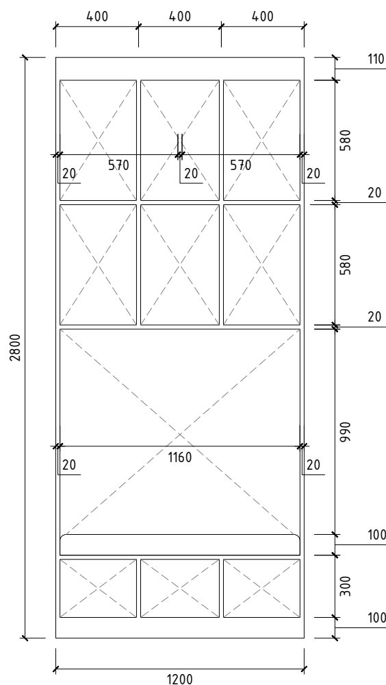
LK 2 - LOKER PENYIMPANAN 2 TAMPAK DEPAN (TERBUKA) SKALA 1 : 25
