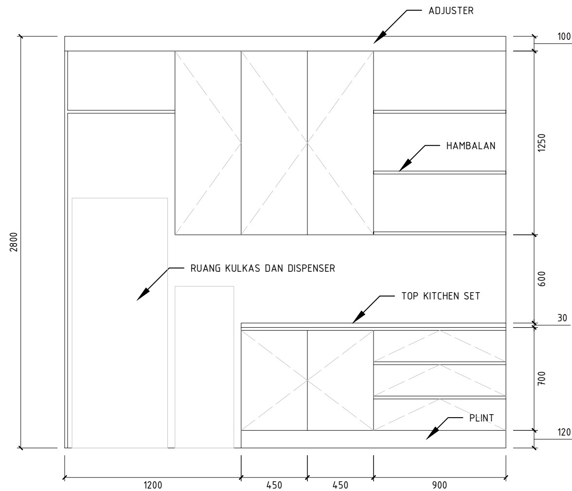
KP - KABINET PANTRY TAMPAK DEPAN SKALA 1 : 25
