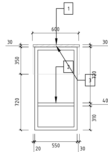
MB - MEJA BAR TAMPAK SAMPING SKALA 1 : 25
