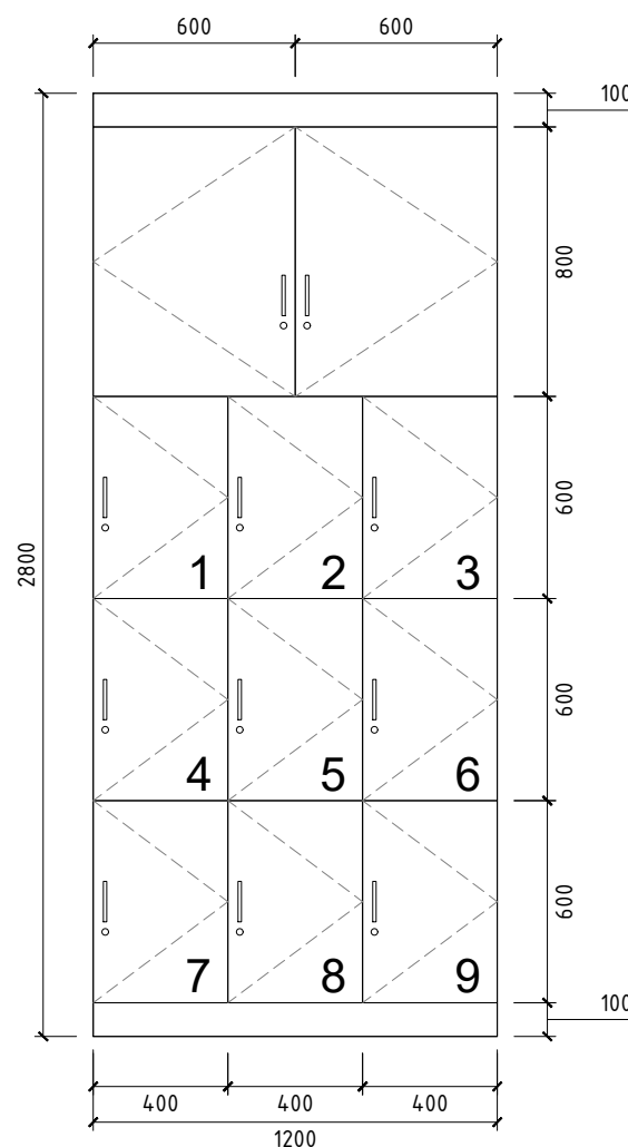
LK 1 – LOKER PENYIMPANAN 1 TAMPAK DEPAN SKALA 1 : 25
