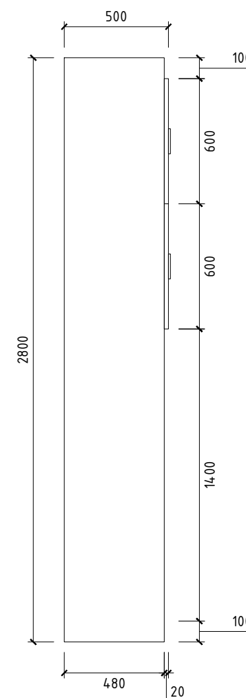
LK 2 - LOKER PENYIMPANAN 2 TAMPAK SAMPIING SKALA 1 : 25
