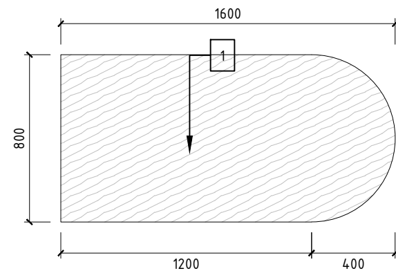
MB - MEJA BAR TAMPAK ATAS SKALA 1 : 25
