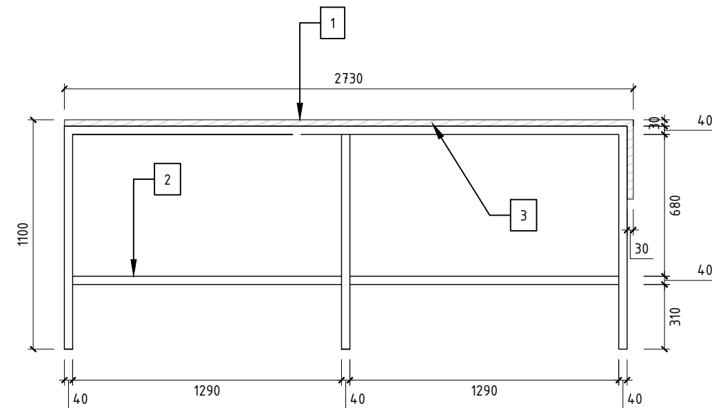
MB - MEJA BAR TAMPAK DEPAN SKALA 1 : 25
