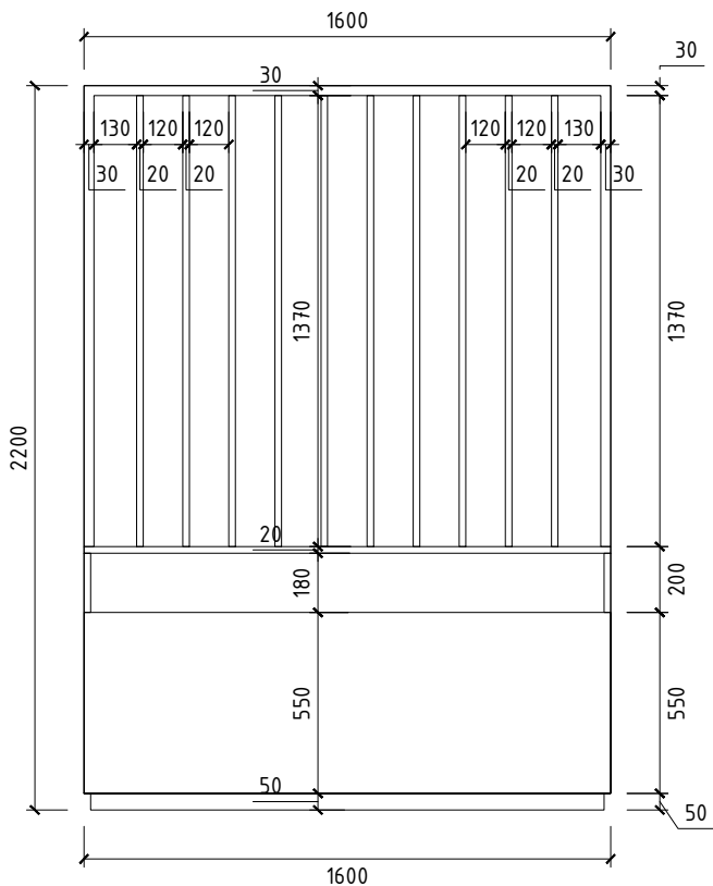
PB - PLANTER BOX TAMPAK DEPAN (TERBUKA) SKALA 1 : 25
