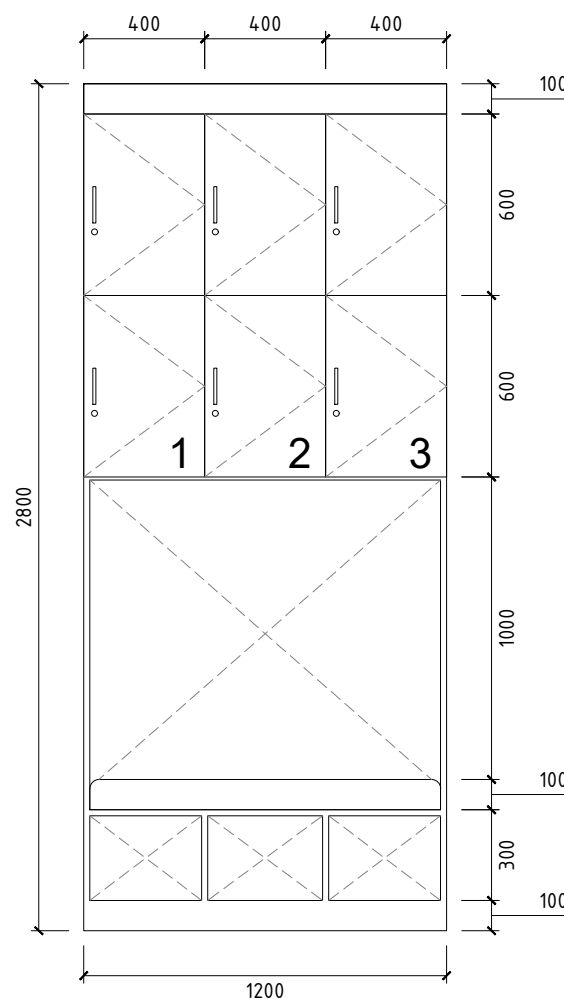
LK 2 - LOKER PENYIMPANAN 2 TAMPAK DEPAN SKALA 1 : 25
